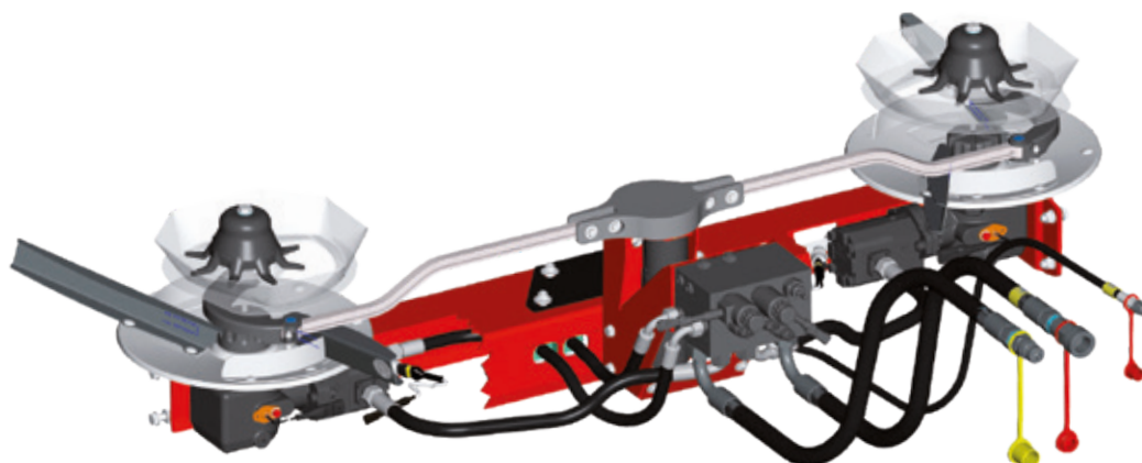
ENTRAÎNEMENT HYDRAULIQUE
